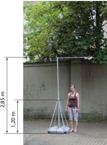
Teleskopmaststellung 1
